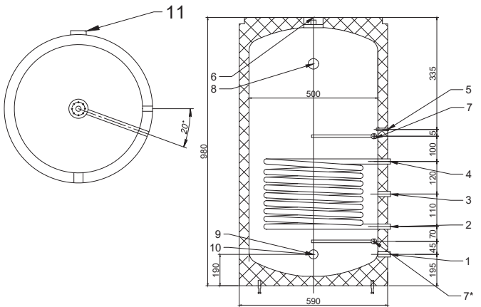
Рис. 1. Размеры SWH-2210-R/L00150
