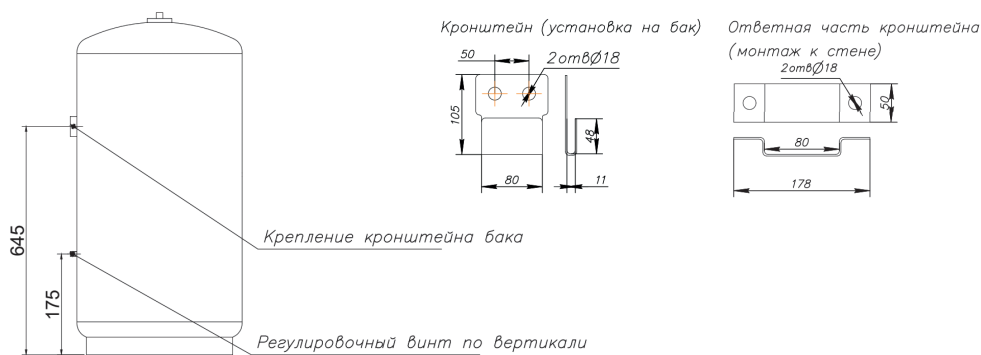
Рис. 4. Конструкция кронштейна настенного крепления
