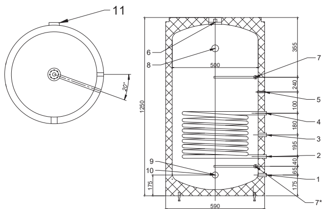
Рис. 2. Размеры SWH-2210-R/L00200
